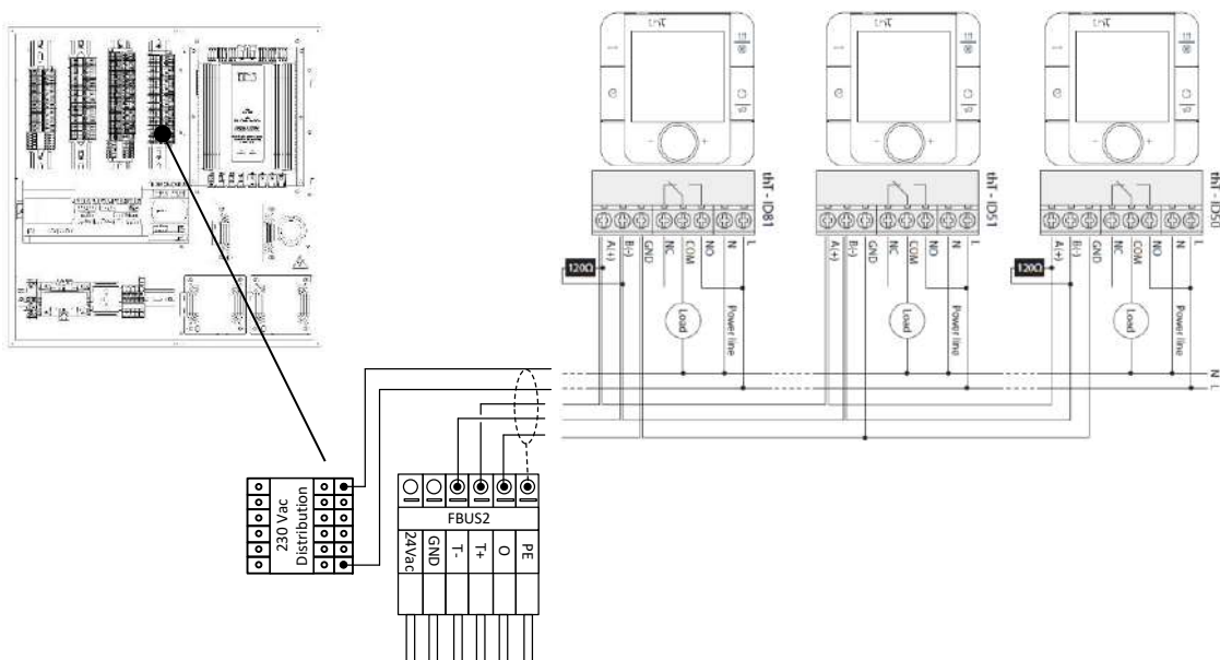
Figure 5.14. Exemple de raccordement d'unités terminales thT
