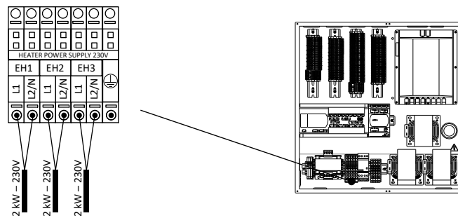
Figure 5.11. Exemple de branchement monophasé avec 2, 4 ou 6 kW
