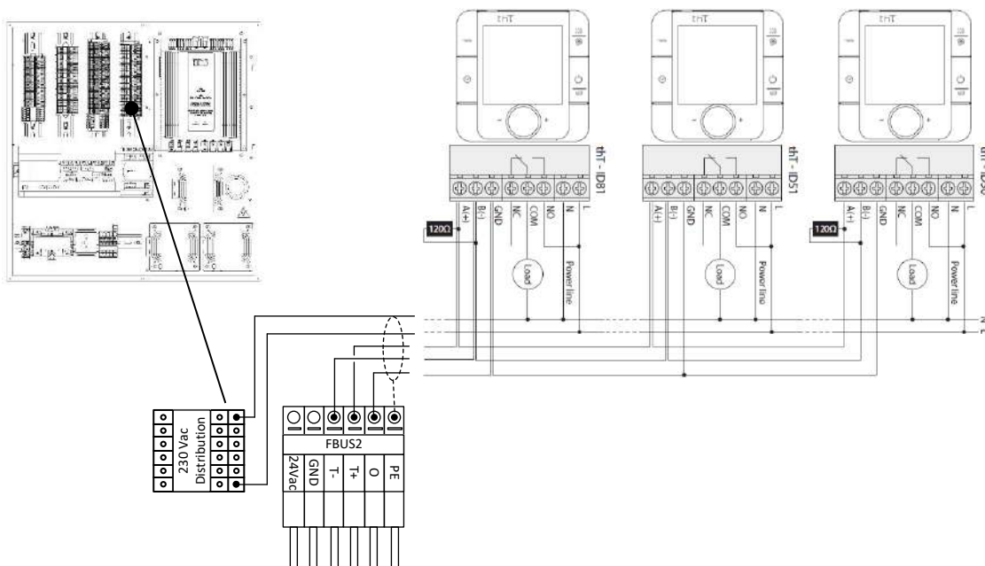
Figura 5.13. Ejemplo de conexión de terminales thT.
